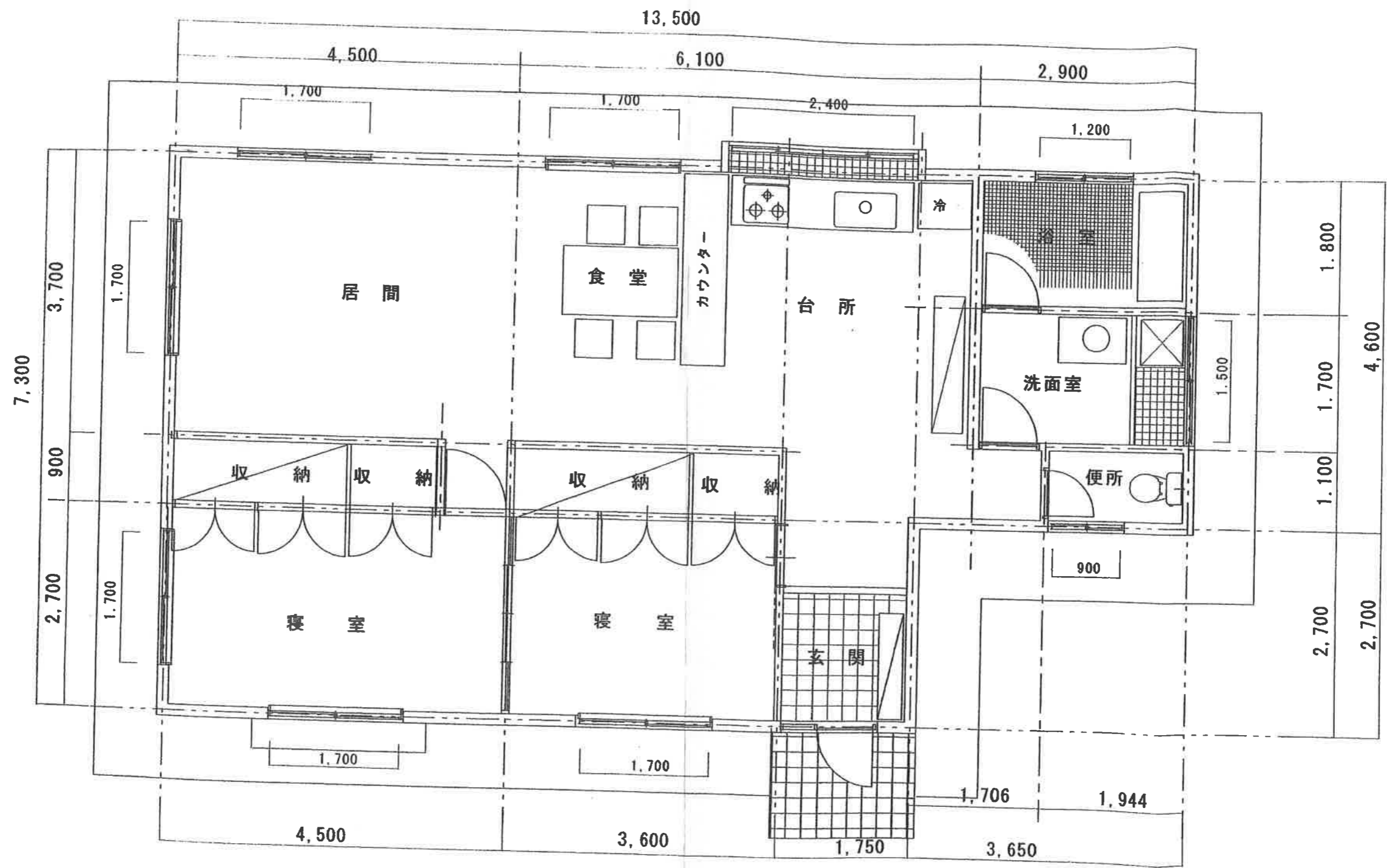
平面図
